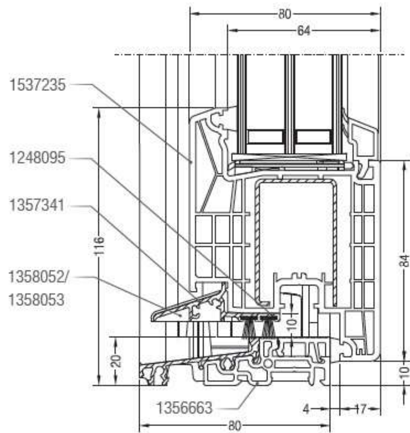
Sezione nodo anta dritta da 85 mm e soglia in Al
