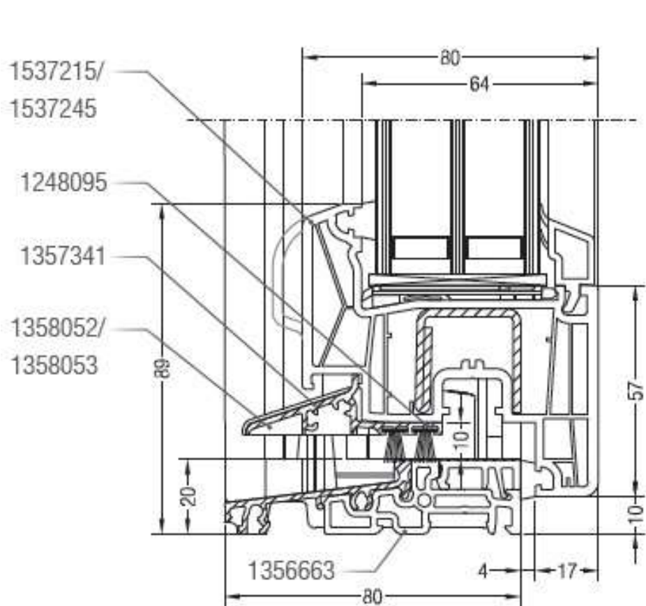
Sezione nodo anta arrotondata/dritta da 57 mm e soglia in Al
